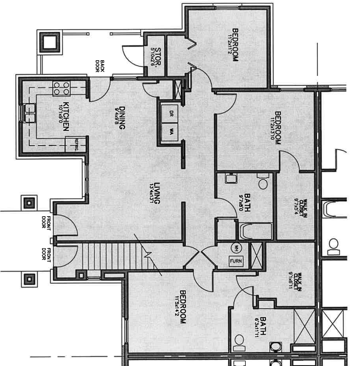
1 TYPE B LOWER H.C. PLAN A4 SCALE: 1/8" = 1'-0"
