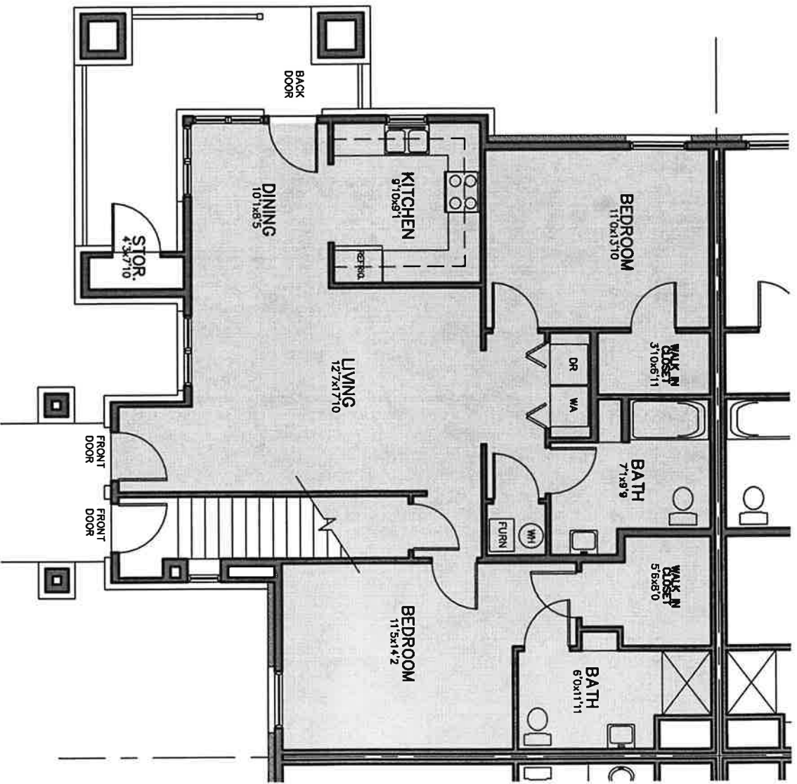
1 TYPE A LOWER H.C. PLAN A3 SCALE: 1/8" = 1'-0"
